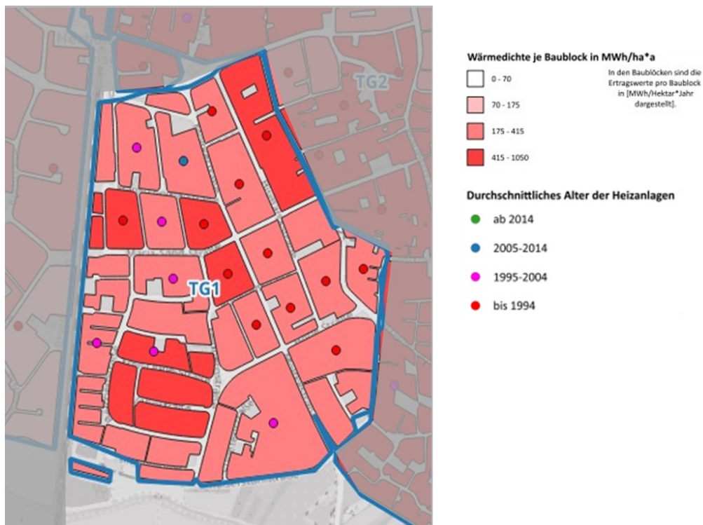
Abbildung 80: Ausschnitt Wärmedichte und Erzeugeralter auf Baublockebene (Ausschnitt Herbolzheim)
